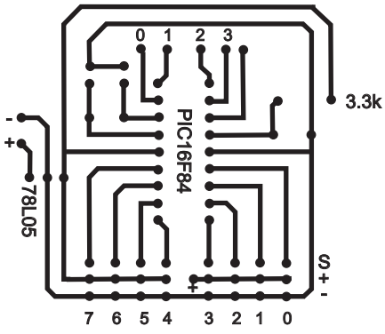
Lado Cobre (abajo)
