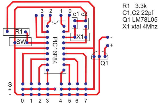
Lado Componentes (arriba)
